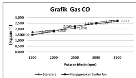
Gambar 3. Gas CO Hasil Pembakaran
