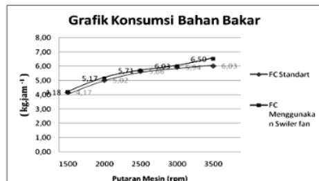
Gambar 2. Konsumsi Bahan Bakar
