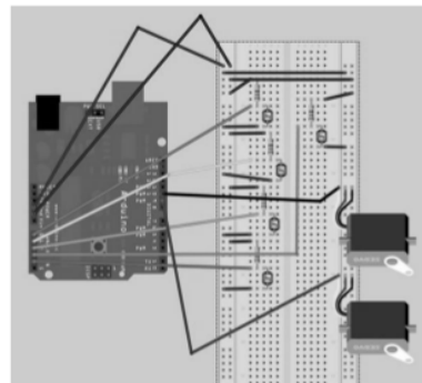
Gambar 3. Rangkaian elektrik Solar Tracker
