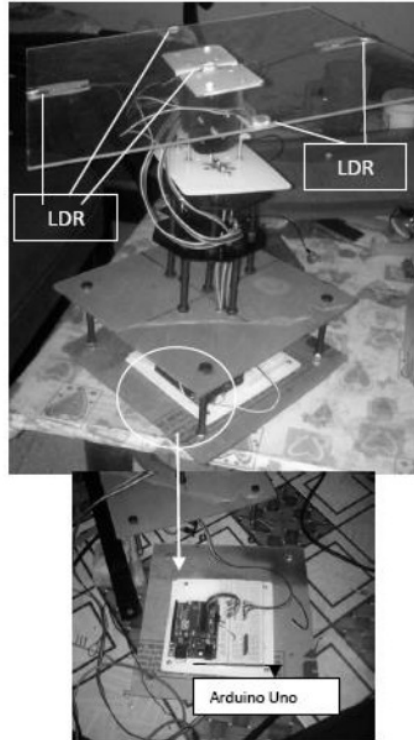
Gambar 5. Posisi Sensor dan Board Arduino
