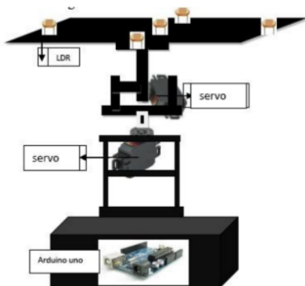
Gambar 2. Rancangan Bangun Solar Tracker
