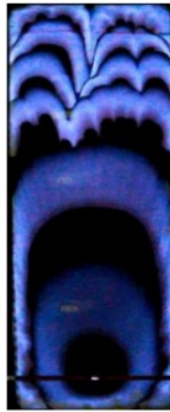
Gambar 3. Pola Rambat Api Campuran Gas Metana-Udara dan N 2 20%
