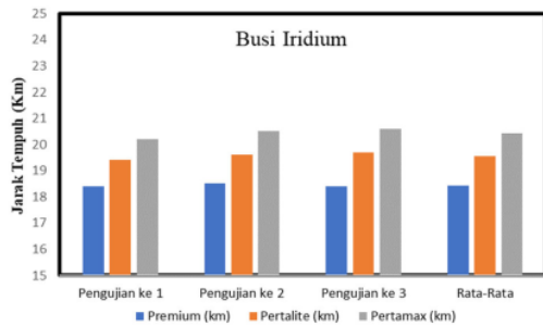
Gambar 5. Pengujian jarak tempuh dengan busi iridium
