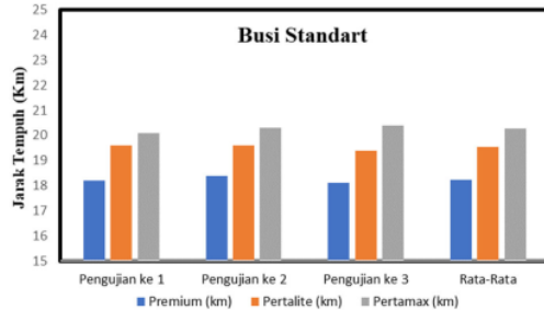
Gambar 4. Pengujian jarak tempuh dengan busi standart
