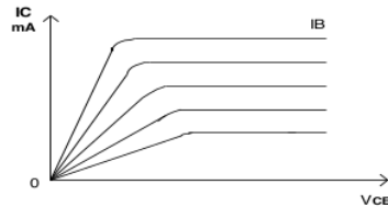
Gambar 6 Grafik Daerah Operasi Transistor Saklar
