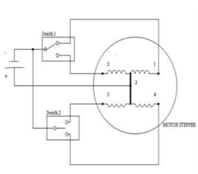
Gambar 10 Rangkaian Pengujian Motor Stepper
