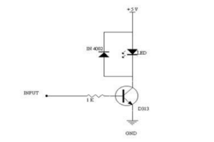
Gambar 9 Rangkaian Pengujian Driver
