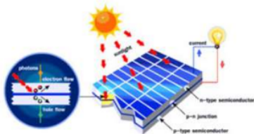
Gambar 2 : Sistem Kerja Solar Cell
