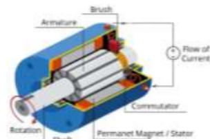
17 Gambar 3 : Motor DC Magnet Permanen
