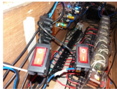
Gambar 11. unit kontrol pada mobil sel surya.
