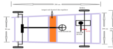
Gambar 7. Mobil sel surya tampak atas
