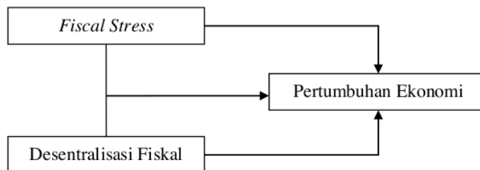
Gambar 1. Kerangka Penelitian
