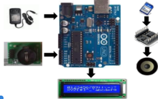
Gambar 2. Desain Perangkat Keras
