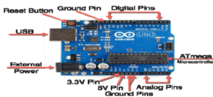
Gambar 1. Arduino Uno
