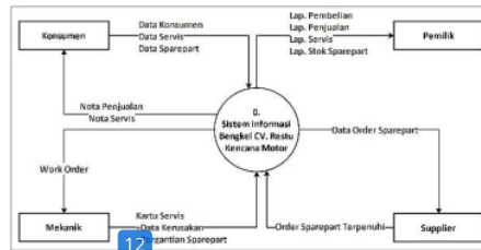
Gambar 3.4 Diagram Konteks
