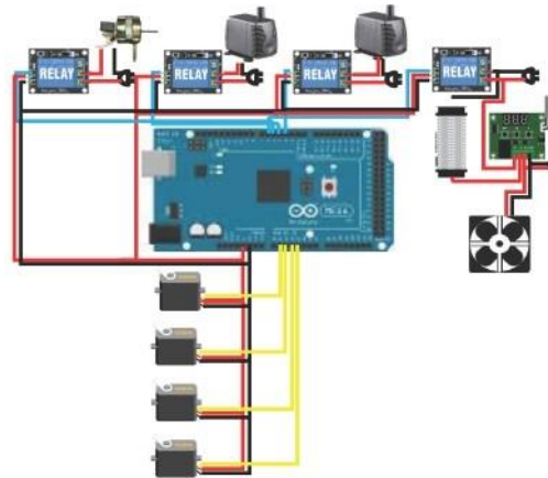
Gambar 11 Rangkaian keseluruhan sistem
