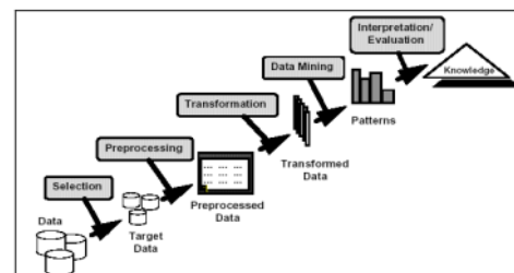
Gambar 1. Tahapan KDD
