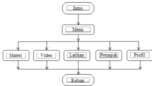
Gambar 3.2 Rancangan Menu Aplikasi
