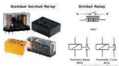
Gambar 3. Bentuk & Simbol Relay
