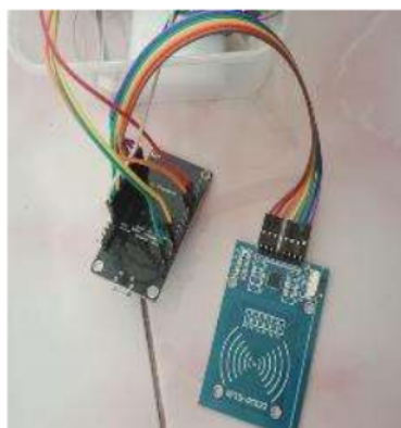
Gambar 11. Rangkaian Sensor RFID dengan ESP8266
