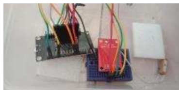
Gambar 12. Rangkaian Modul GPS Neo-6M
