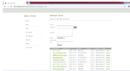
Gambar 4.7 Menu siswa
