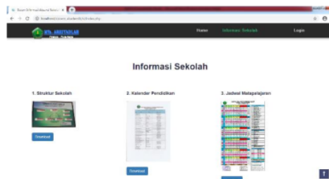
Gambar 4.2 Informasi Sekolah
