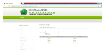
Gambar 4.6 Menu Kelas
