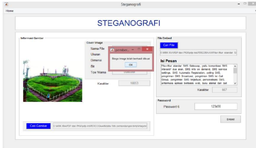
Gambar 6 : Proses Encode
