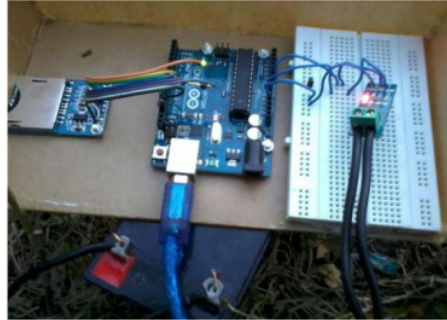
Gambar 3. Foto Data Logger
