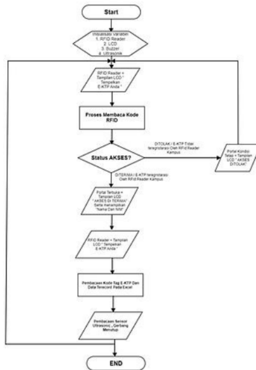
Gambar 5. Langkah-langkah Sistem Perancangan Miniatur Parkir
