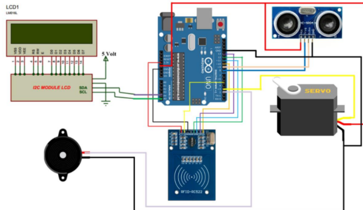
Gambar 1. Skematik Rangkaian Sistem
