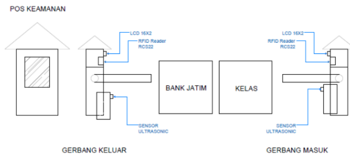
Gambar 8. Miniatur Mekanisme Palang Parkir
