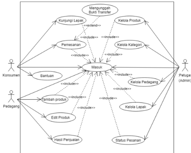
Gambar 2. Use Case Diagram Pemesanan
