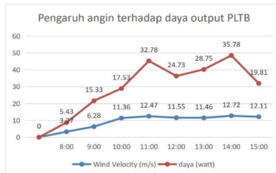
Gambar 9. Grafik pengaruh kecepatan angin terhadap daya output PLTB
