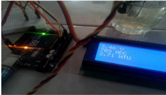
Gambar 3.4 sensor kekeruhan pada air bening
