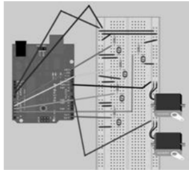
Gambar 3. Rangkaian elektrik Solar Tracker
