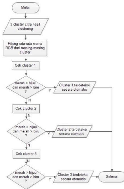
Gambar 2. Flowchart deteksi otomatis
