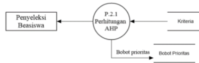
Gambar 10. DFD Level 2
