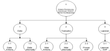
Gambar 6. Diagram Berjenjang
