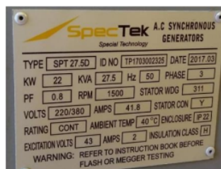
Gambar 4. Plate Spesifikasi Turbin
