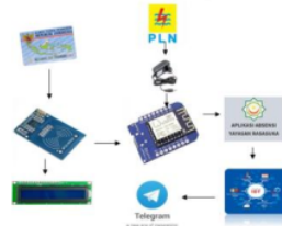
Gambar 12. Desain Perangkat Presensi
