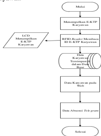
Gambar13. Algoritma RFID pada Presensi Karyawan
