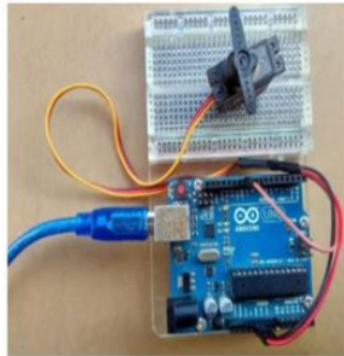
Gambar 3. Rangkaian Motor Servo
