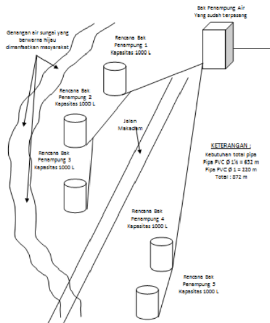
Gambar 4. Peta Jaringan Pipanisasi pada 5 Tandon Air
