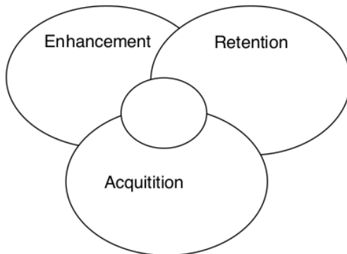
Gambar 2. Siklus CRM
